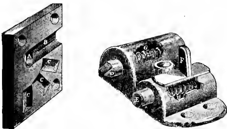
Fig. 4397. Ratchet-plate.
